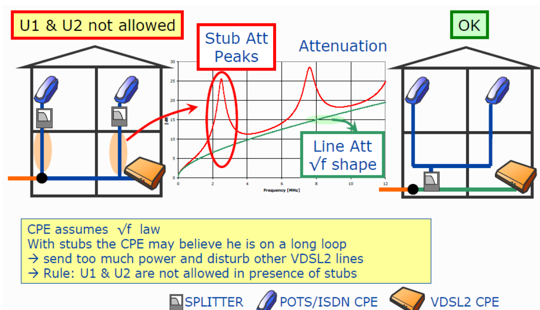
Figuur: Interne bekabeling bij de eindgebruiker
