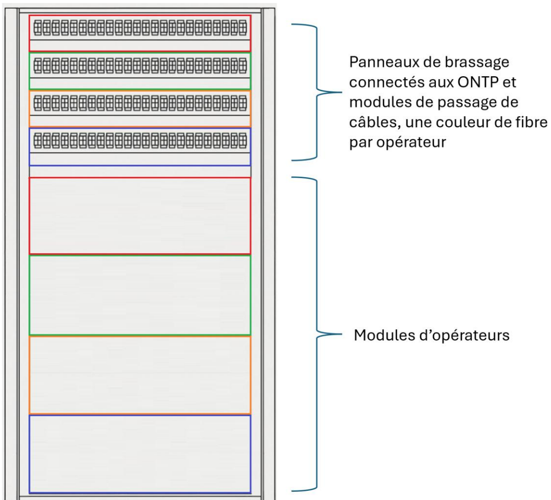
Figure 7 : Schéma d'ODF
