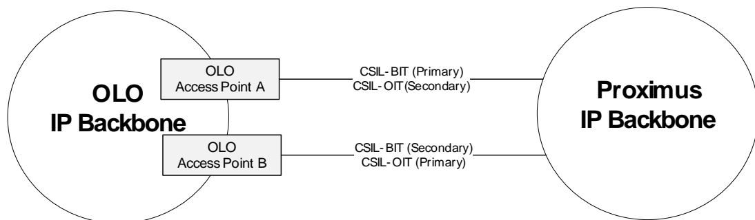
Figuur 2: architectuur waarbij de OLO niet aanwezig is op de toegangspunten van Proximus
