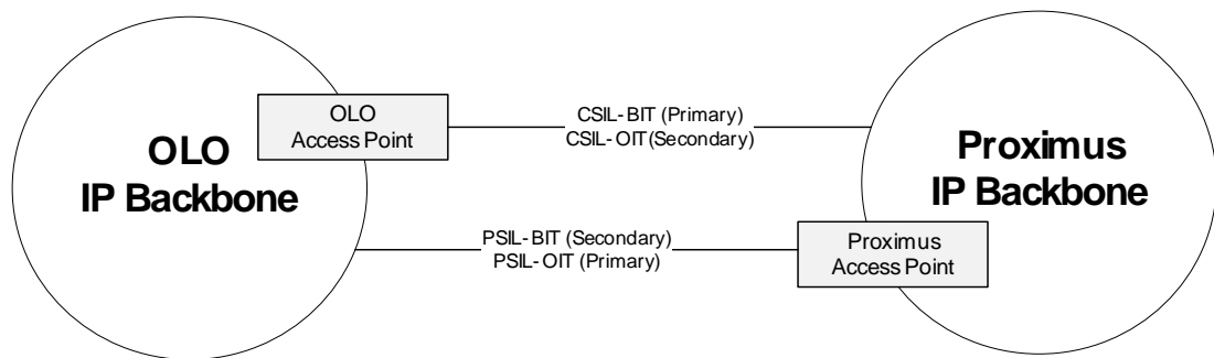
Figuur 3: architectuur waarin de OLO slechts aanwezig is op één toegangspunt van Proximus
